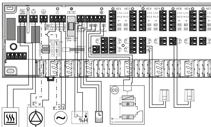
Obr. 67. Elektrické sběrnice Basic+ 230 V nebo 24 V.
