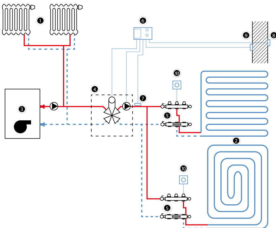
Obr. 52. S c h é m a centrálního systému směšování s automatickou regulací
