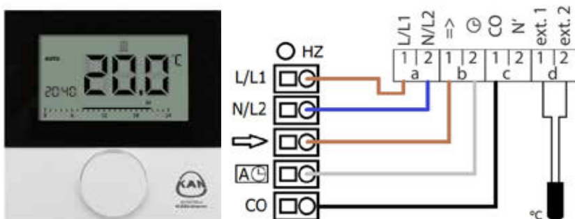
Obr. 70. Schéma svorek a připojení termostatu Basic+ s LCD Control topení/chlazení, 230 V nebo 24 V (s možností řízení celou automatiku s využitím vnitřních hodin).
