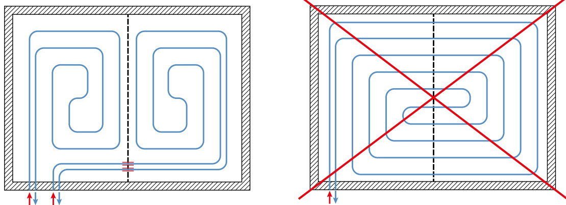
Obr. 19. Správné a chybné rozdělení otopné plochy dilatační spárou
