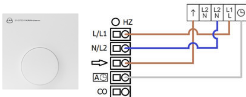
Obr. 64. Schéma svorek a připojení čidla teploty s nastavením Basic+ 230 V nebo 24 V k elektrické sběrnici Basic+ (s možností dočasného snížení teploty pomocí připojení hodin).
