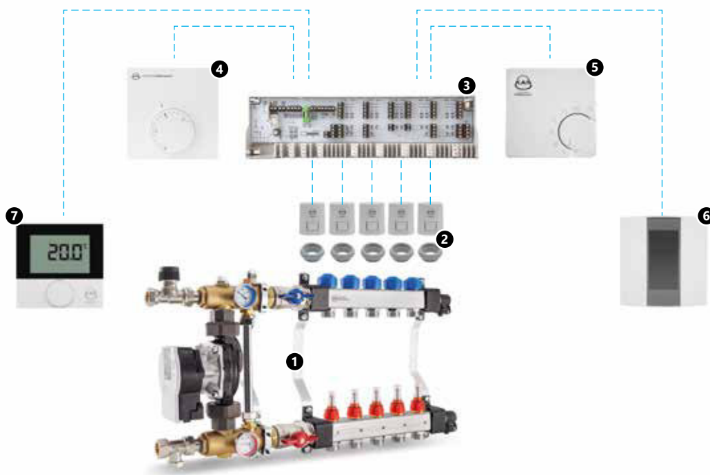
Obr. 61. Příklad lokálního nastavení vedení a automatiky KAN-therm v plošném vytápění.
