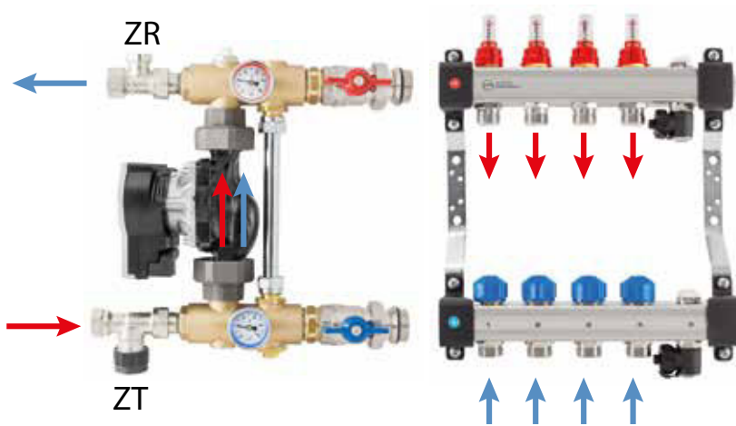
Obr. 59. Čerpadlová skupina se stálými hodnotami s rozdělovačem UFST – směry průtoků.
