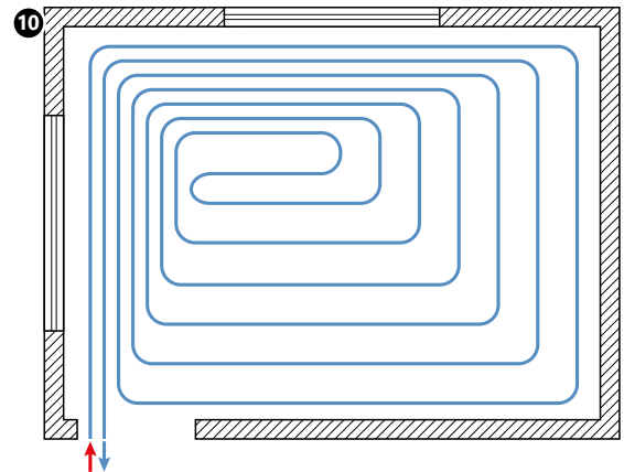
Obr. 10. Potrubí podlahového vytápění/chlazení se spirálovým uložením, s okrajovou zónou provedenou z jedné smyčky položené podél obvodových stěn nebo ploch s velkými otvorovými výplněmi.
