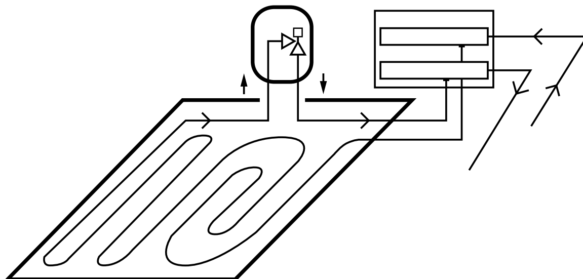
Obr. 77. Schéma fungování – skupina umístěná na vratném potrubí
