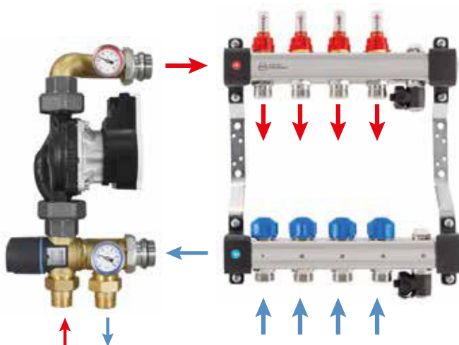
Obr. 60. Čerpadlová skupina s termostatickým třicestným směšovacím ventilem UFST – směry průtoků.
