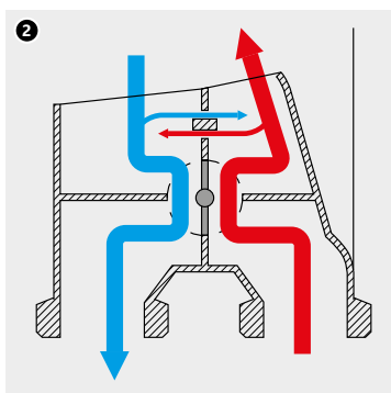
1. Směšovač KAN-Bloc s čtyřcestným ventilem v tepelně izolačním plášti 2. Princip fungování čtyřcestného ventilu ve směšovači KAN-Bloc
