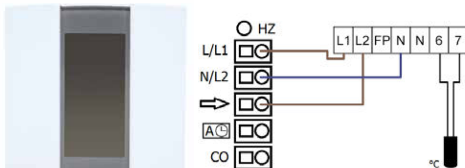
Obr. 68. Schéma svorek a připojení týdenního termostatu TH232-AF.
